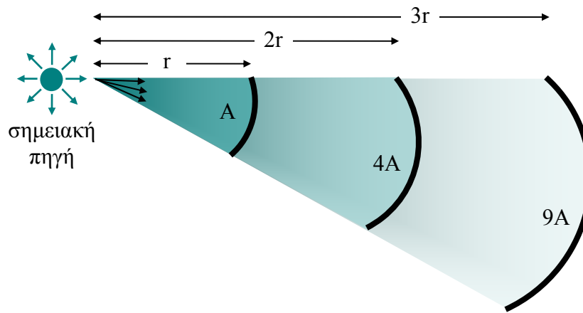
Σχήμα 7. Σχηματική παράσταση του φωτομετρικού νόμου των αποστάσεων. Η φωτεινή ροή που αναδύεται από σημειακή πηγή μέσα σε στερεά γωνία, κατανέμεται σε όλο και μεγαλύτερες επιφάνειες, με αποτέλεσμα ο φωτισμός να μειώνεται αντιστρόφως ανάλογα με το τετράγωνο της απόστασης.
