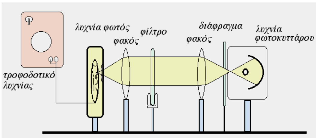
Σχήμα 5.: Σχηματική παράσταση του οπτικού μέρους της πειραματικής διάταξης
