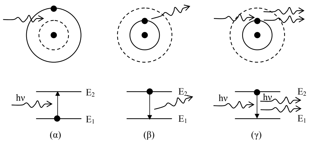
Σχήμα 4. (α) Εξαναγκασμένη απορρόφηση. (β) Αυθόρμητη εκπομπή. (γ) Εξαναγκασμένη εκπομπή (παραγωγή Laser).
