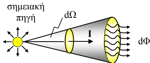
Σχήμα 2. Φωτοβολία σημειακής πηγής
