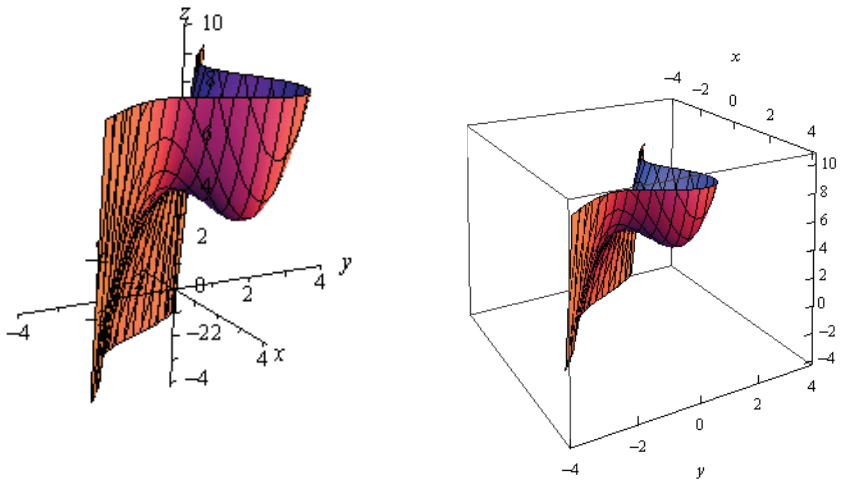
Σχήμα 4.3.1 - 3: Παράδειγμα 4.3.1 - 3. Δύο διαφορετικές όψεις του διαγράμματος της f(x, y) = x^3 + y^3 - 3xy + 4
