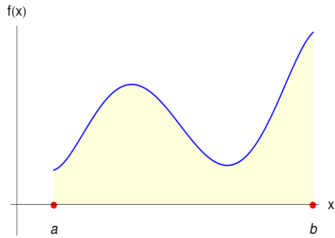
Σχήμα 7.1.1 - 1: γεωμετρική ερμηνεία του ορισμένου ολοκληρώματος \int_a^b f(x) dx
