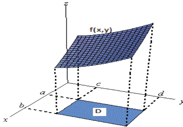
Σχήμα 7.1.1 - 2: γεωμετρική ερμηνεία του διπλού ολοκληρώματος \iint_D f(x,y) dx dy
