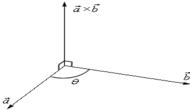
Σχήμα 5.1 - 5: εξωτερικό γινόμενο των διανυσμάτων \alpha και \beta
