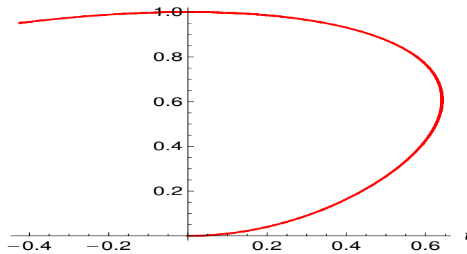
Σχήμα 5.1 - 6: Παράδειγμα 5.1 - 4: η καμπύλη με παραμετρική εξίσωση \mathbf{F}(t) = \sqrt{t} \cos t \mathbf{i} + \sin t \mathbf{j} , όταν t \in [0, 3\pi/5]
