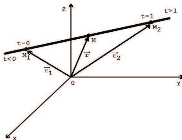
Σχήμα 5.2 - 3: Παράδειγμα 5.2 - 1: παραμετρική παράσταση του ευθύγραμμου τμήματος M_1M_2
