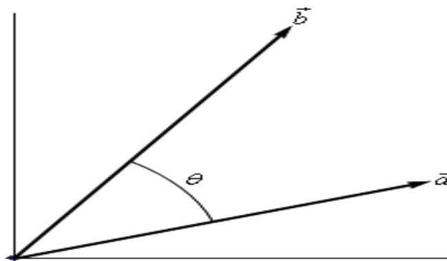
Σχήμα 5.1 - 4: εσωτερικό γινόμενο των διανυσμάτων \alpha και \beta
