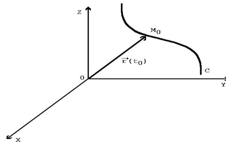
Σχήμα 5.2 - 1: παραμετρική παράσταση καμπυλών
