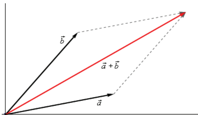
Σχήμα 5.1 - 3: πρόσθεση διανυσμάτων
