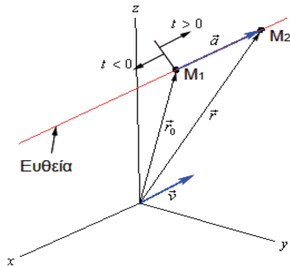
Σχήμα 5.2 - 2: παραμετρική παράσταση ευθείας
